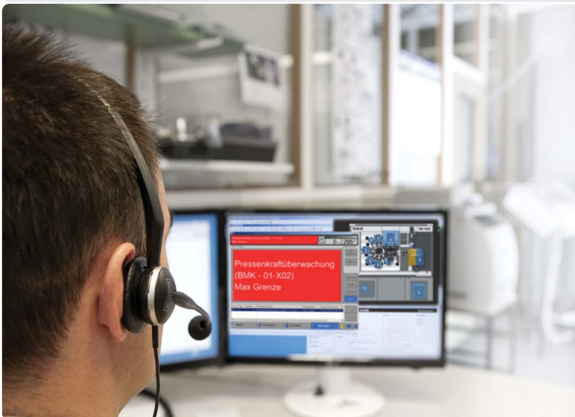
Bild 1: Virtuell vor Ort: das Teleservice-Portal gibt dem Techniker Fernzugriff auf Visualisierung, Steuerung und alle weiteren netzwerkfähigen Komponenten einer Maschine.
